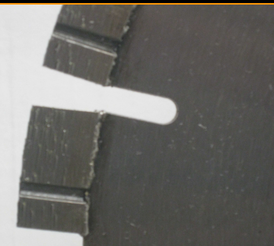
esempio di disco con segmento alto 10 mm turbo - sample of disc with segment height 10 mm turbo
