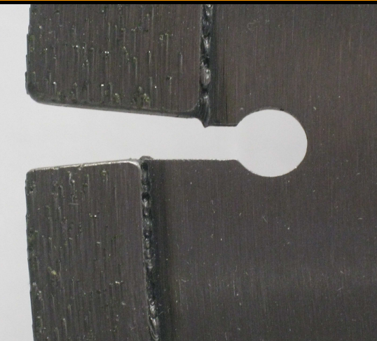
esempio di disco con segmento alto 10 mm + drop - sample of disc with segment height 10 mm + drop
